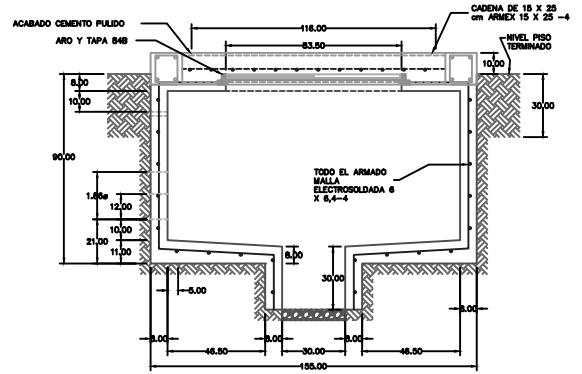
NIVEL FREÁTICO BAJO CORTE B-B
