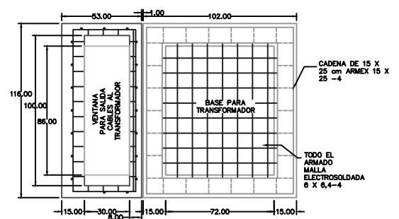
PLANTA BASE PARA TRANSFORMADOR CUANDO SE FABRICA INDEPENDIENTE DEL REGISTRO
